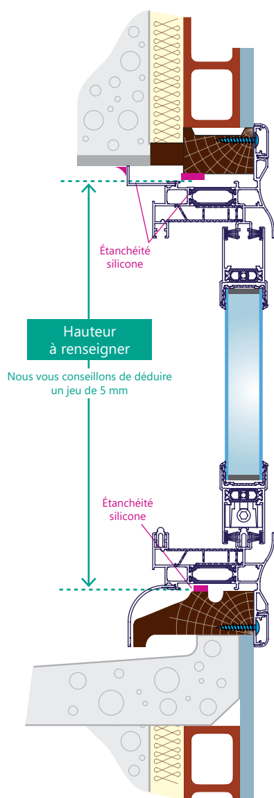
Fig 2. Coupe verticale
