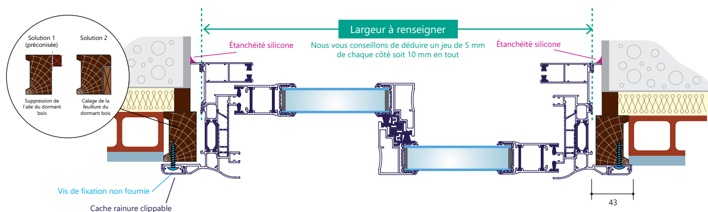
Fig 5. Coupe horizontale
