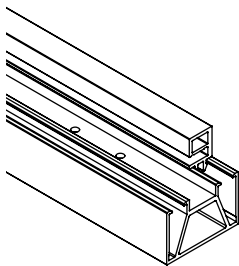
Traverse H/B
