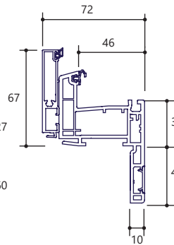
Rénovation fixation façade
