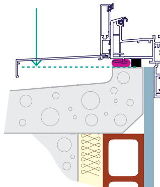
Fig 14. Variante avec suppression de l'appui en bois
