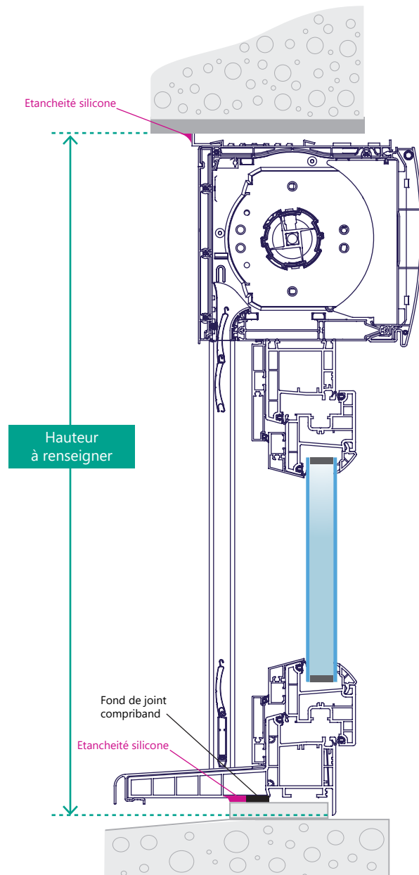
Fig 32. Coupe verticale avec volet roulant
