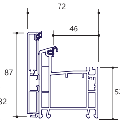
Neuf / Applique sans isolation
