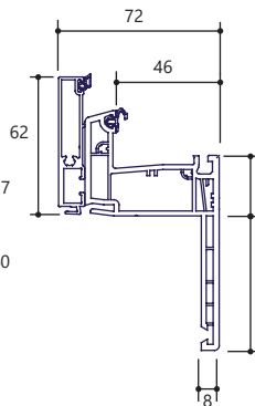
Fenêtre et Porte-fenêtre crémonne (poignée intérieure)
