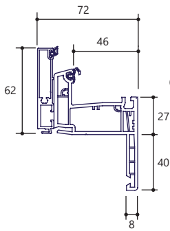
Rénovation aile de 40 mm
