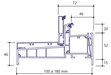
Neuf / Applique avec isolation
