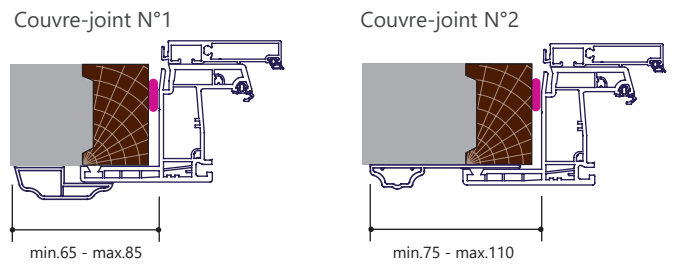
Fig 3. Moulure(s) intérieure(s) rapportée(s) (option)
