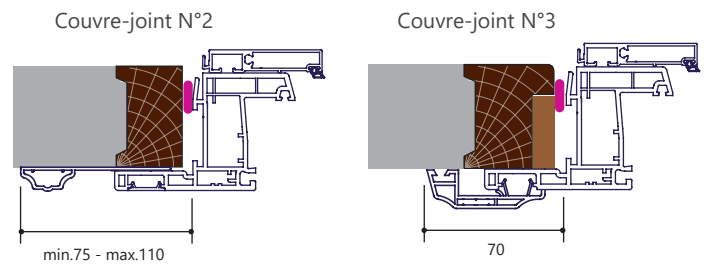
Fig 13. Moulure(s) intérieure(s) rapportée(s) (option)
