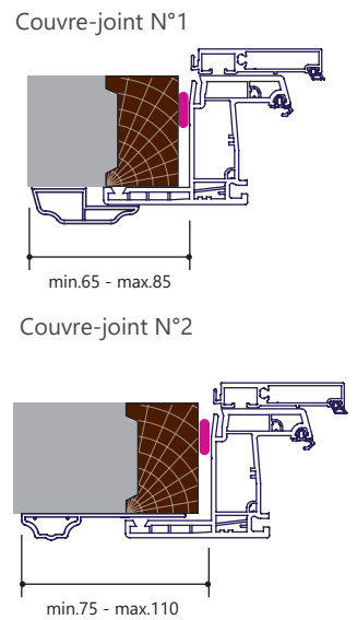
Fig 9. Moulure(s) intérieure(s) rapportée(s) (option)
