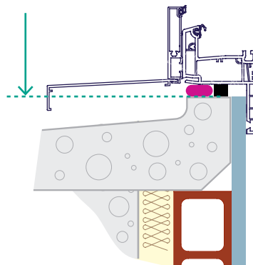
Fig 4. Variante avec suppression de l'appui en bois
