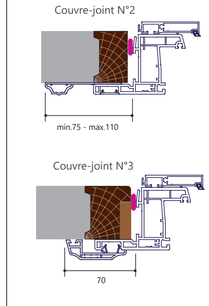
Fig 19. Moulure(s) intérieure(s) rapportée(s) (option)
