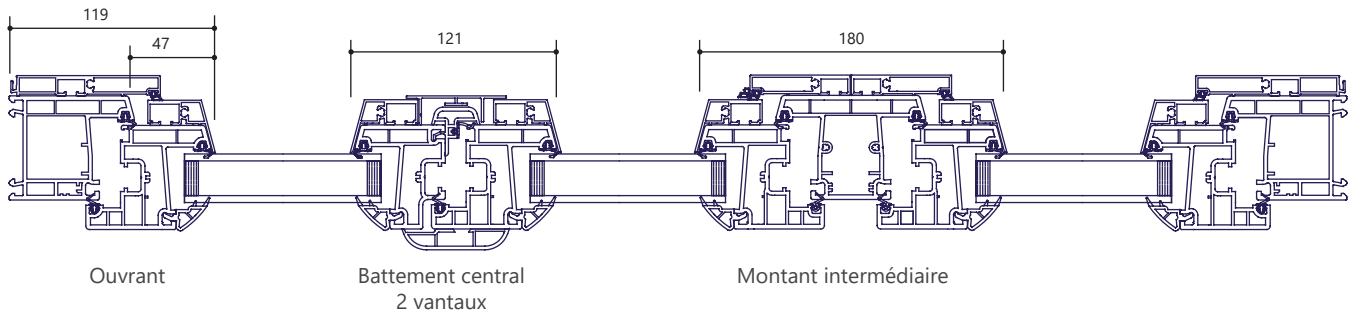
Fenêtre et Porte-fenêtre crémonne (poignée intérieure)
