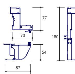
Isolation de 180
