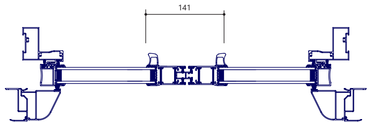
Baies coulissantes 2 vantaux - monorail dormant de 140 à 200 mm
