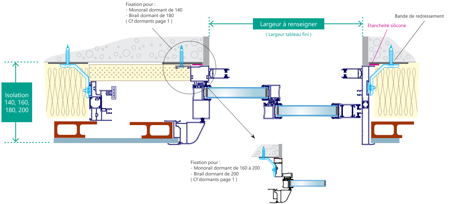
Fig6. Coupe horizontale
