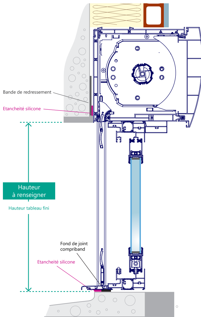
Fig 5. Coupe verticale
