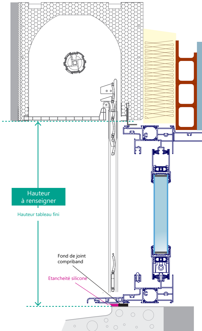
Fig 7. Coupe verticale
