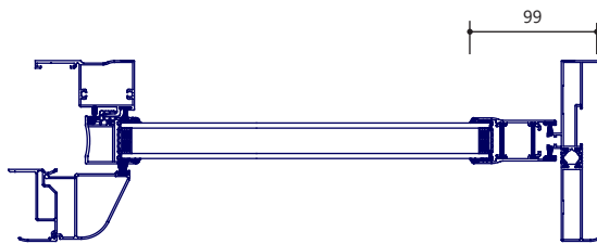
Baies coulissantes 1 vantail - monorail dormant de 140 à 200 mm
