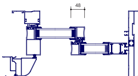
Baies coulissantes 2 vantaux - birail dormant de 180 à 200 mm
