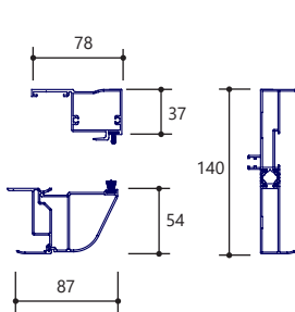
Isolation de 140
