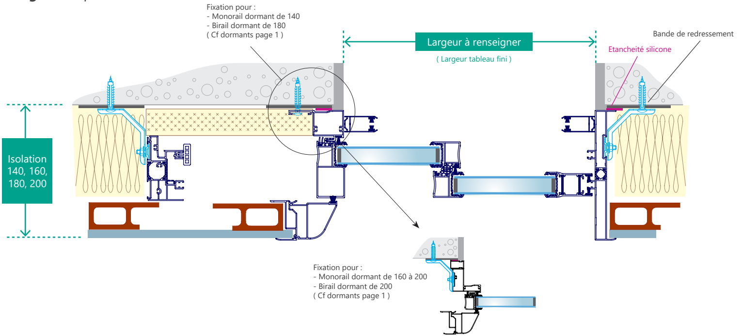
Fig 4. Coupe horizontale
