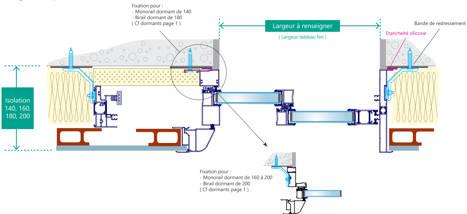
Fig 1. Coupe horizontale
