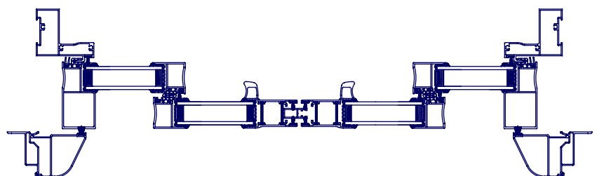
Baies coulissantes 4 vantaux - birail dormant de 180 à 200 mm
