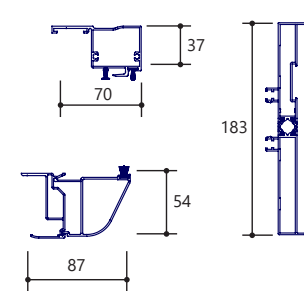
Baies coulissantes 2 vantaux - monorail dormant de 140 à 200 mm
